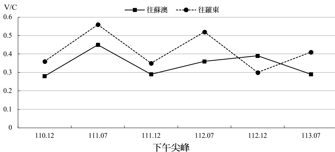
圖2.5-4 台九線歷次尖峰小時PCU變化圖
