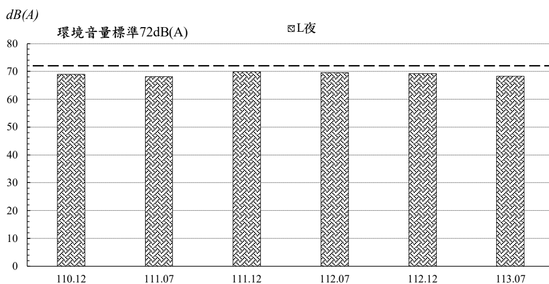
圖2.3-2 台九線噪音監測值與標準比較圖
