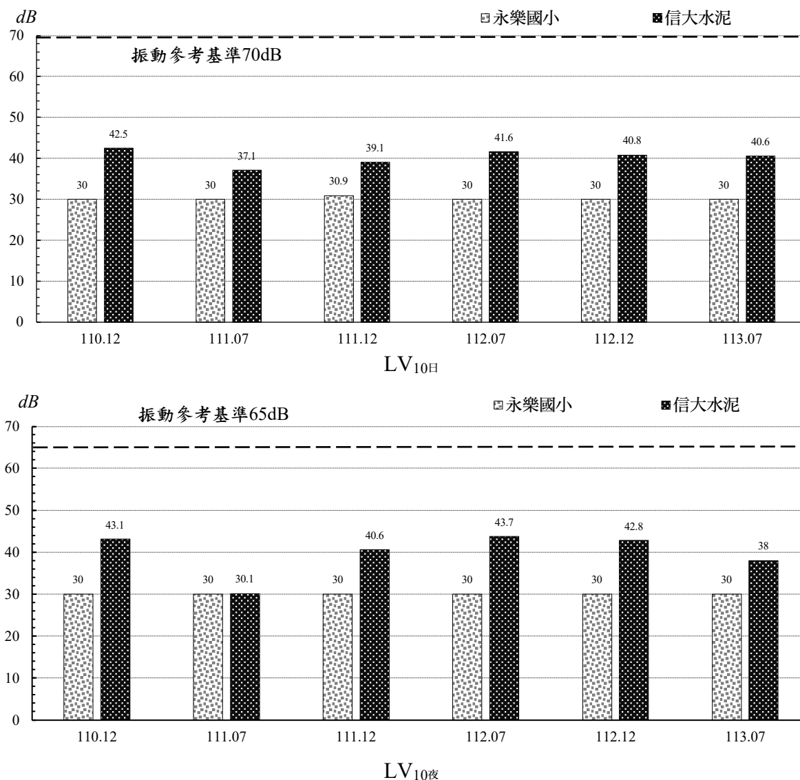
圖2.4-1 振動長時間監測值與參考值比較圖
