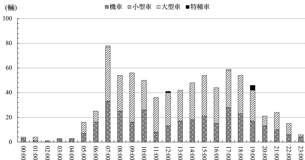
圖2.5-1 永樂路24小時單位車輛組織柱狀圖
