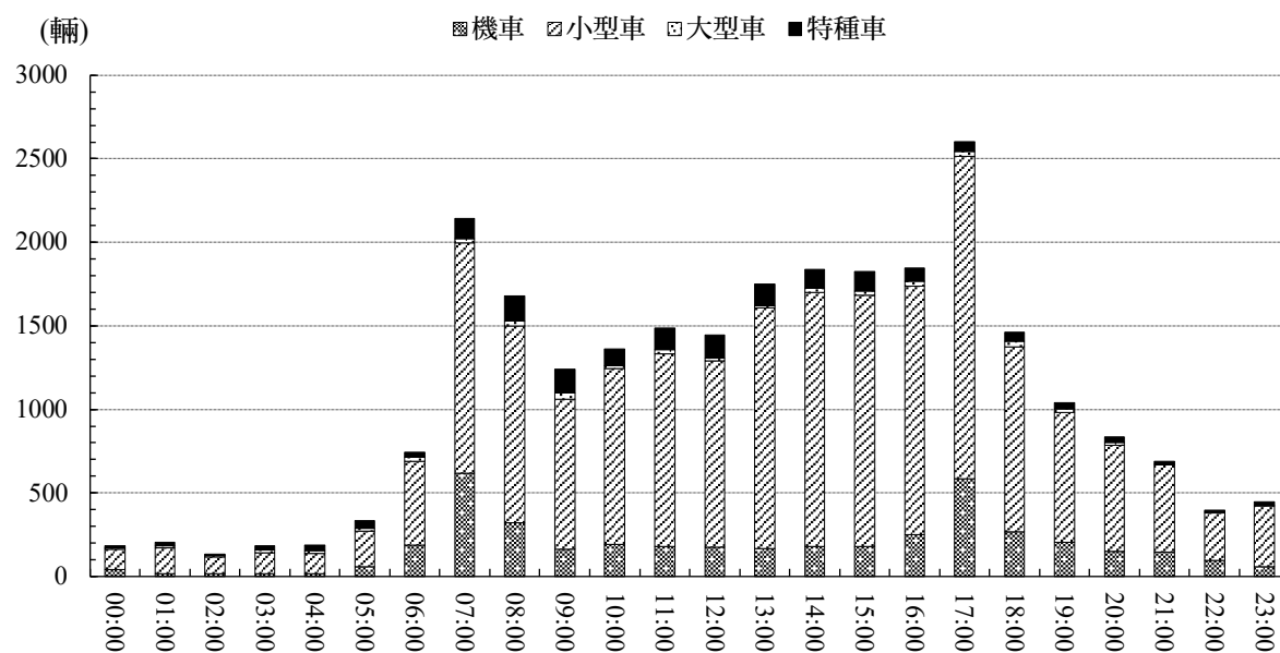
圖2.5-3 台九線24小時單位車輛組織柱狀圖
