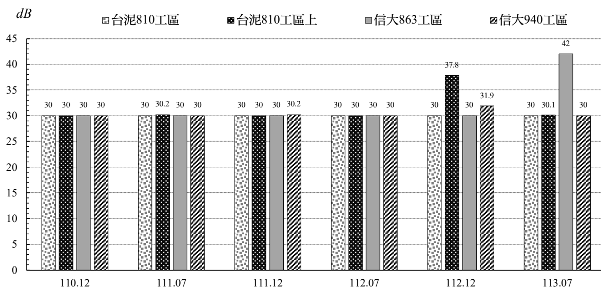
圖2.4-3 礦區四周短時間振動監測結果比較圖
