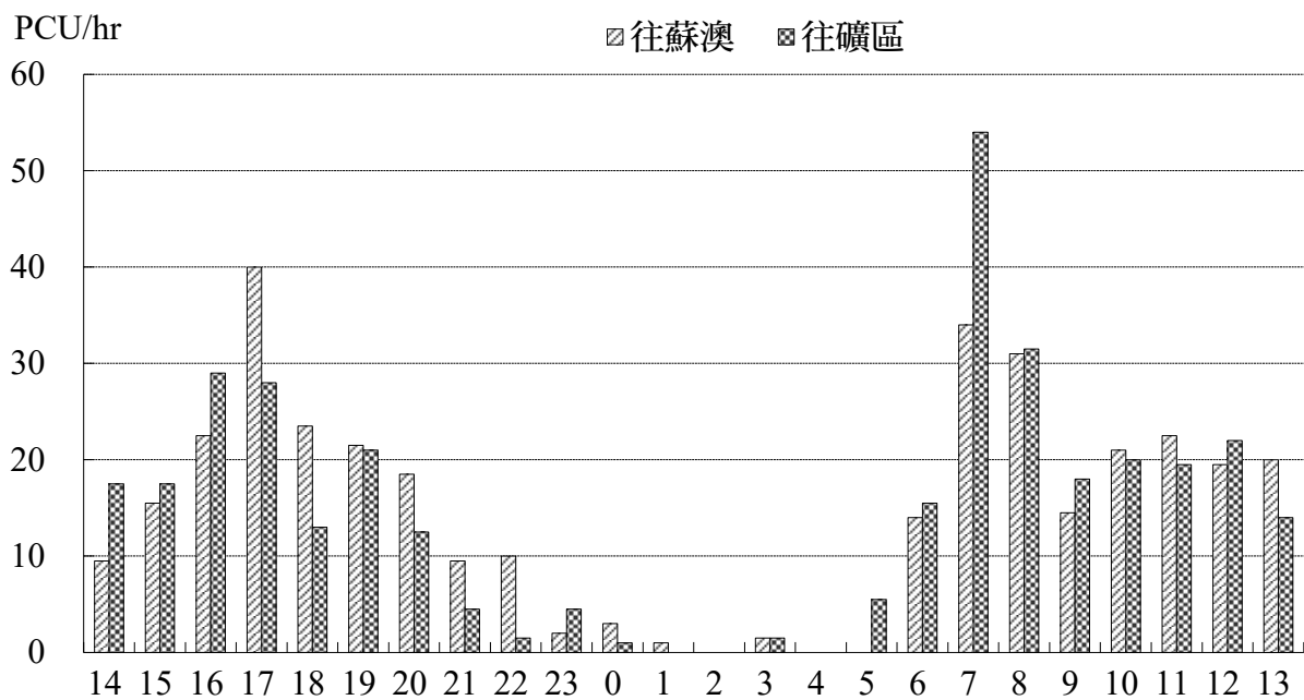
圖2.5-2 永樂路尖峰小時PCU比較圖
