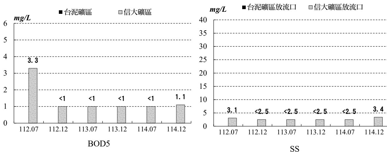
圖2.1-2 放流口地表水水質監測結果圖
