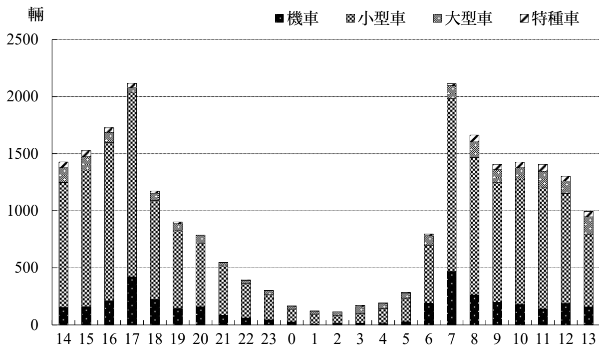
圖 2.5-3 台九線 24 小時單位車輛組織柱狀圖
