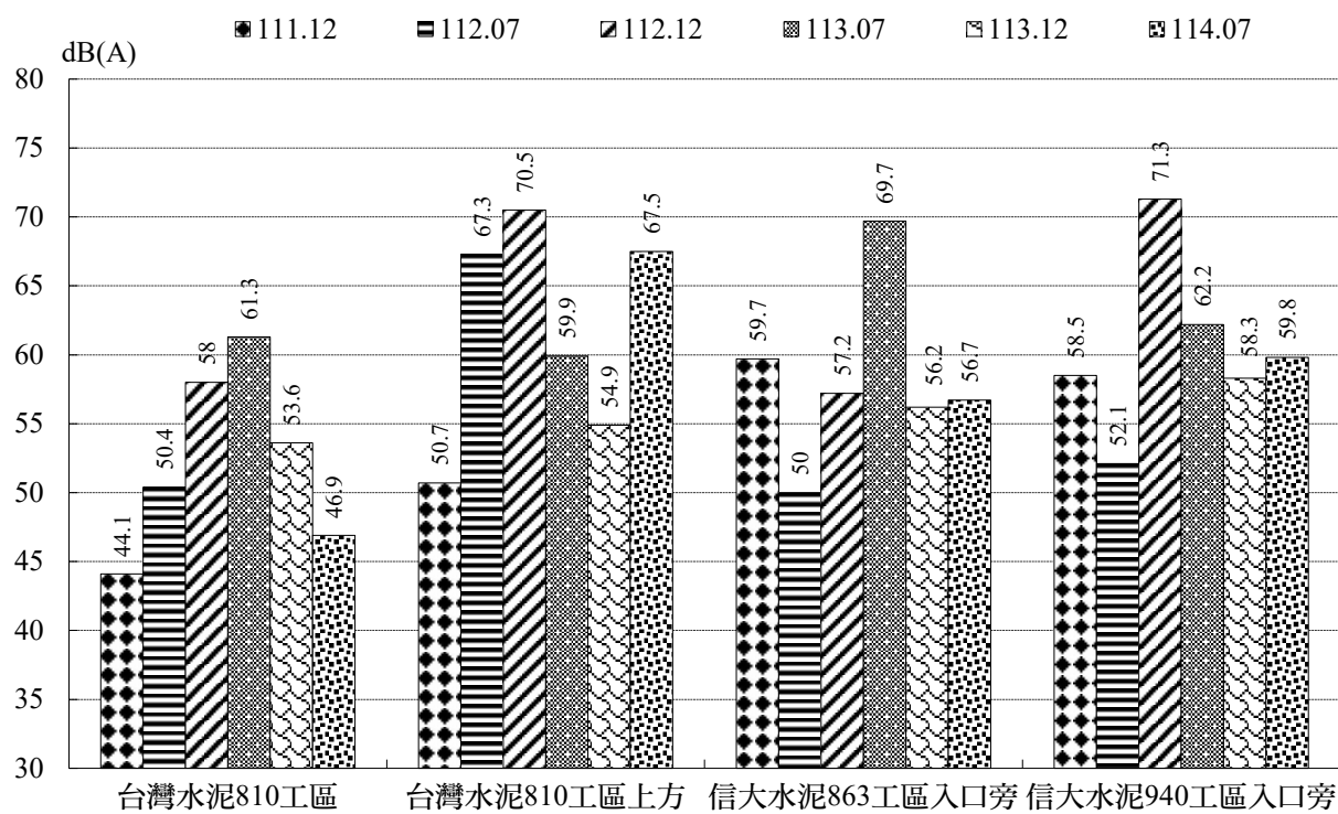
圖2.3-3 均能音量( L_{eq} )與前季之比較圖—計畫場址週界四點
