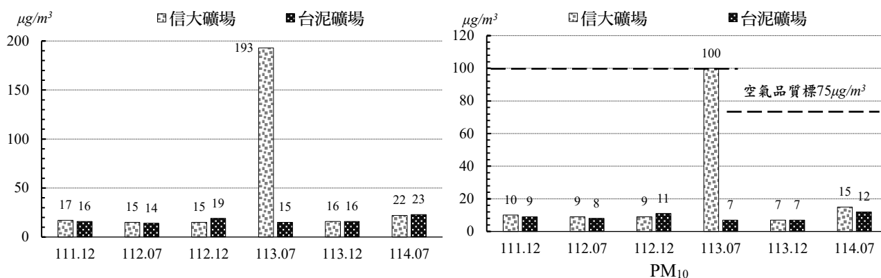
圖2.2-1 信大台泥空氣品質與標準值比較圖
