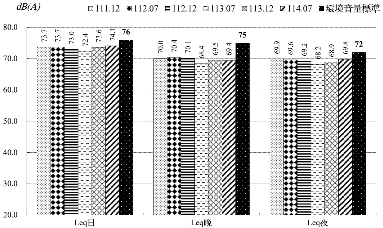
圖2.3-2 台九線噪音監測值與標準比較圖
