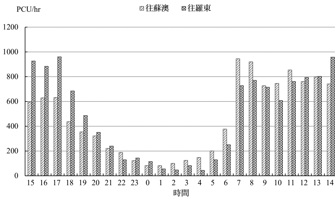
圖2.5-4 台九線尖峰小時PCU比較圖
