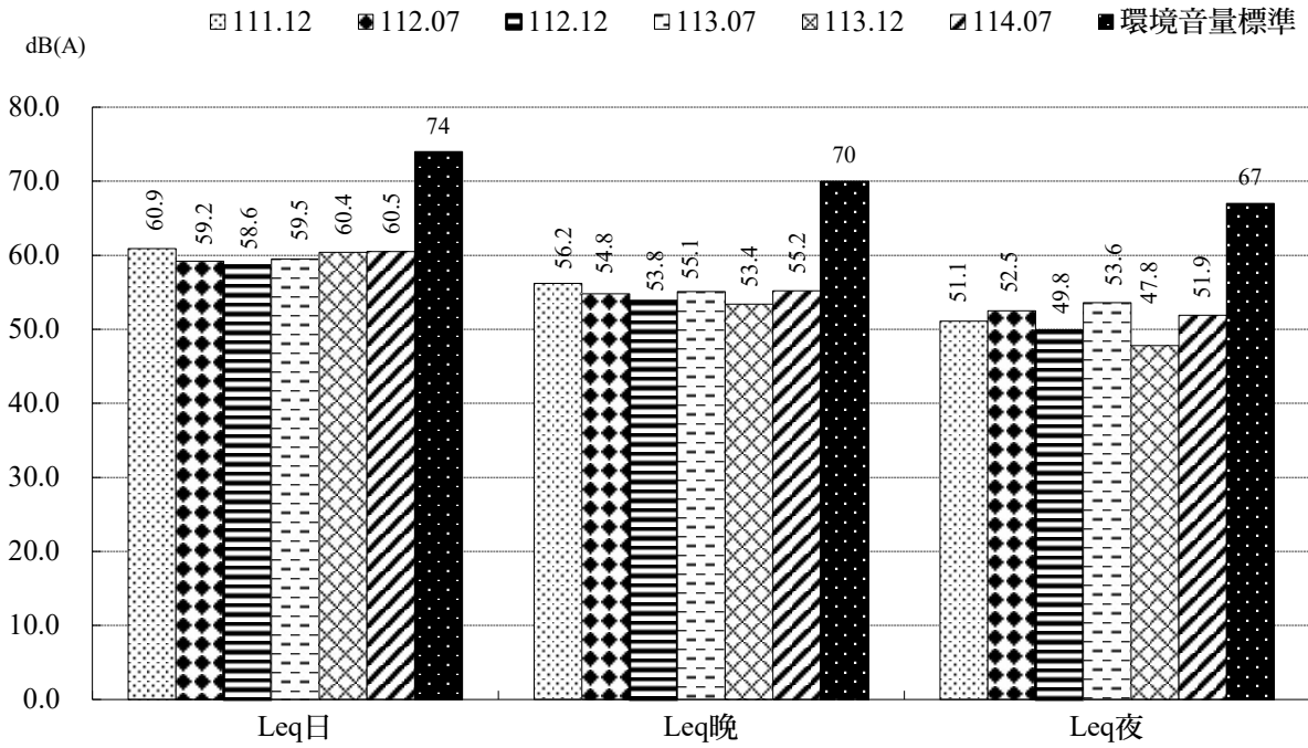
圖2.3-1 永樂路噪音監測值與標準比較圖
