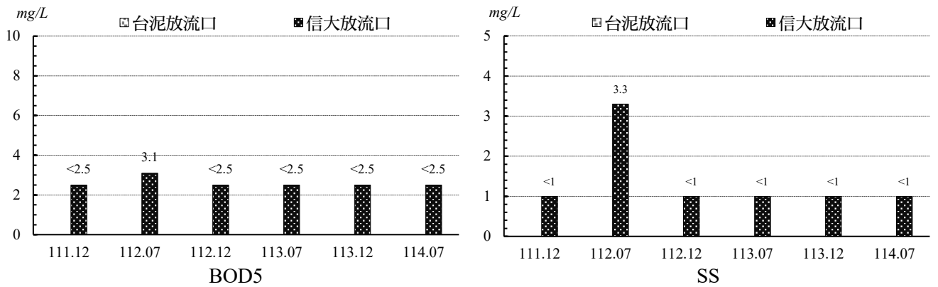
圖2.1-2 放流口地表水水質監測結果圖
