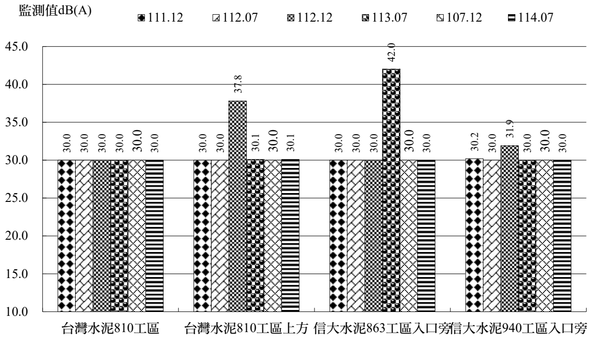
圖2.4-3 礦區四周短時間振動監測結果比較圖
