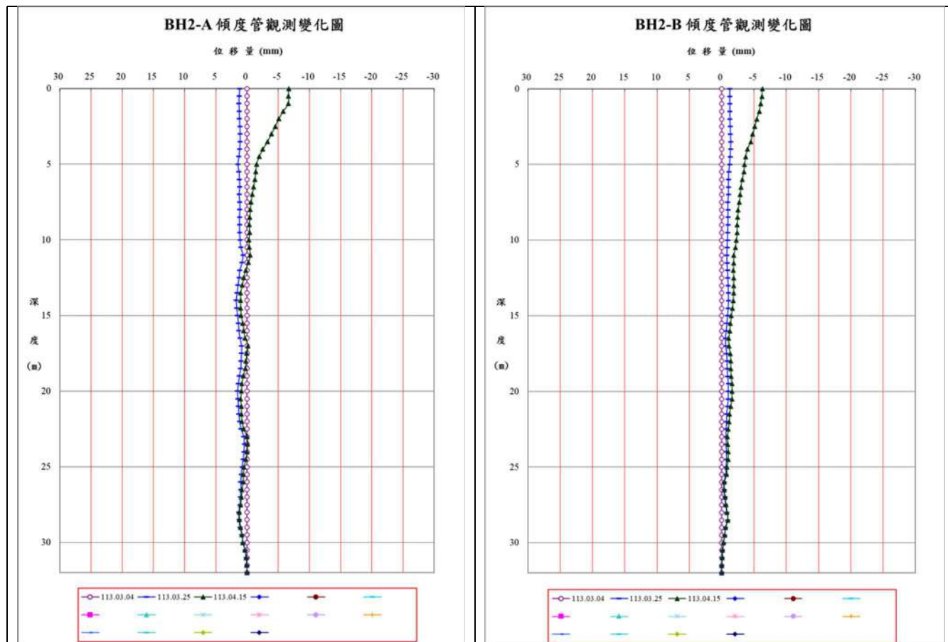
圖8、BH2傾斜管位移曲線（113年3月4日為初始值）
