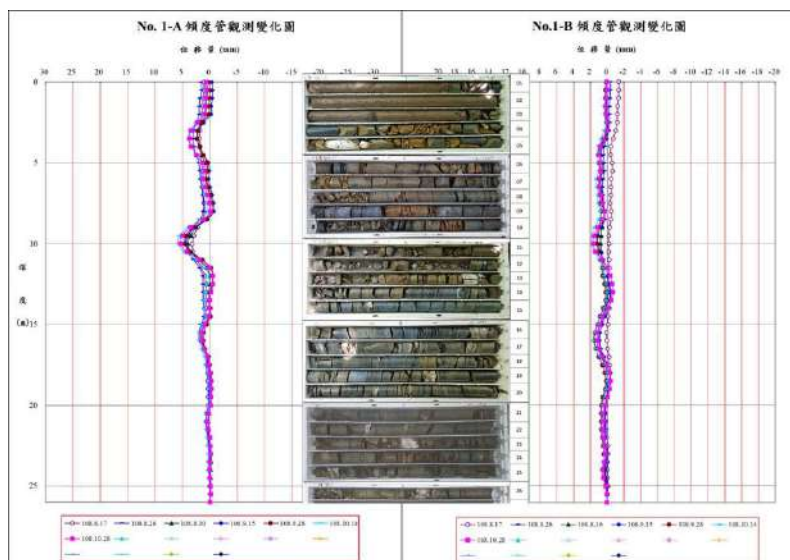
圖2、傾斜管量測情形
