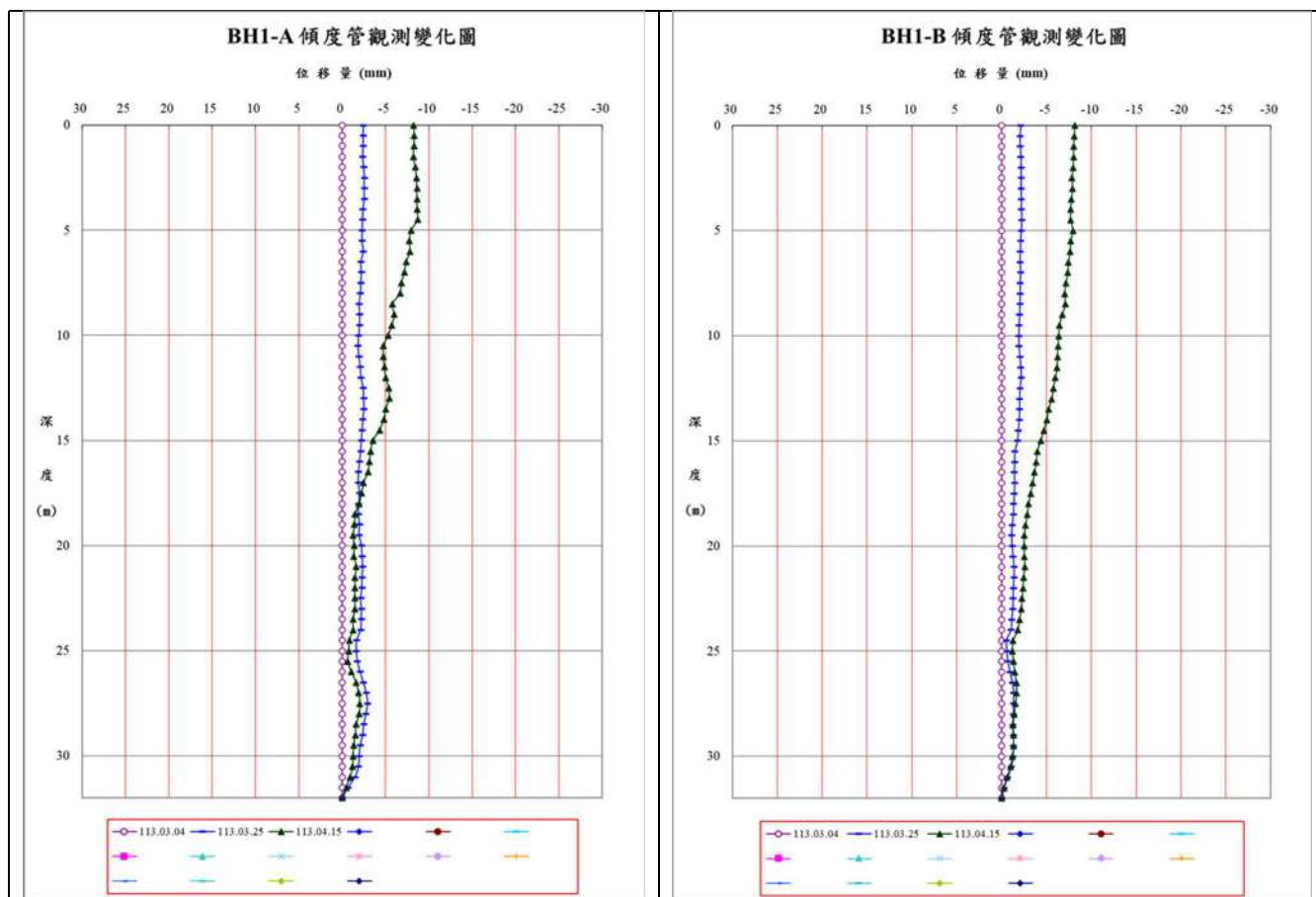
圖7、BH1傾斜管位移曲線（以113年3月4日初始值）
