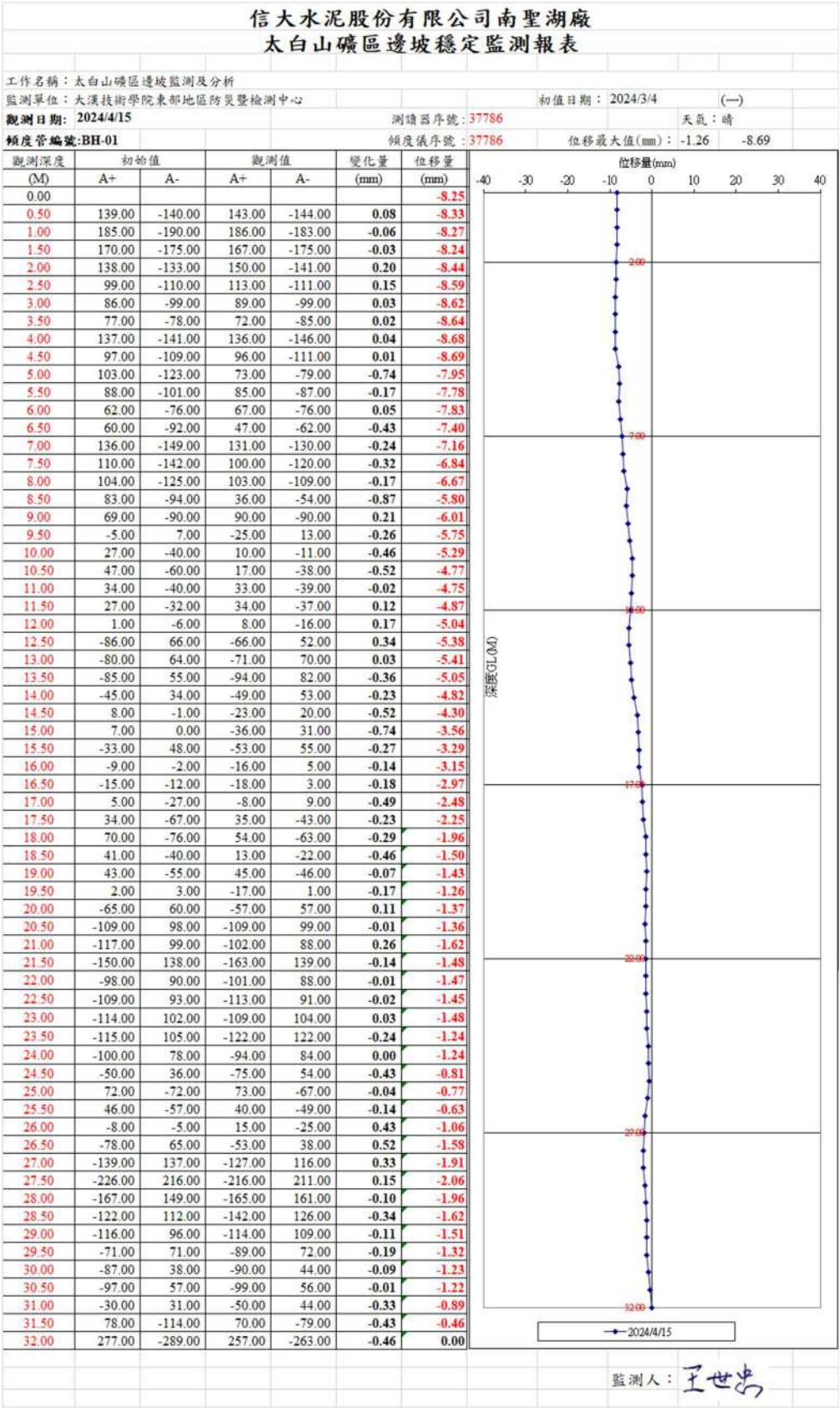
附表一 BH.01~02 傾斜管觀測記錄表（113 年 4 月 15 日，初值日期 3 月 4 日）
