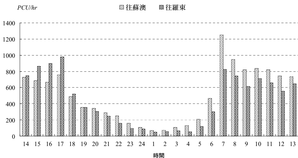
圖2.5-4 台九線尖峰小時PCU比較圖
