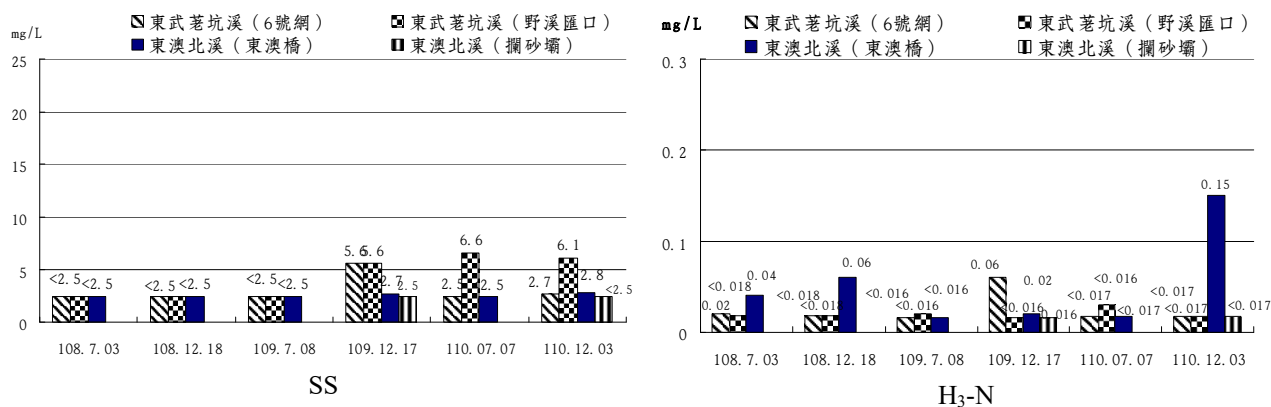
圖2.1-1 東澳北溪、東武荖坑溪地表水水質監測結果圖(續)
