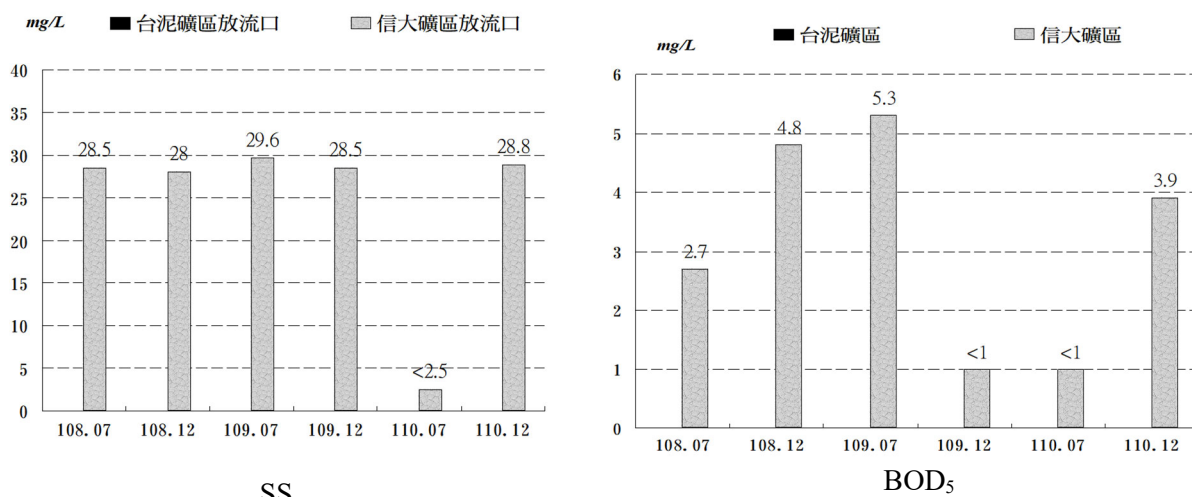
圖2.1-2 放流口地表水水質監測結果圖
