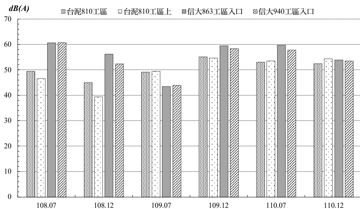
圖2.3-2 均能音量( L_{eq} )與前季之比較圖—計畫場址週界四點
