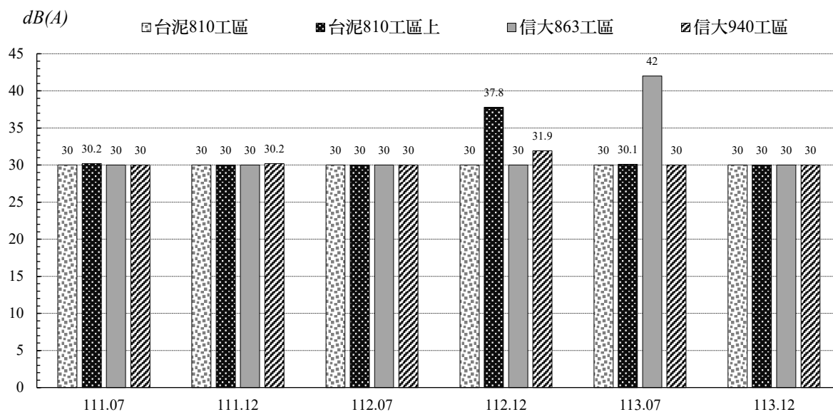
圖2.4-2 礦區四周短時間振動監測結果比較圖
