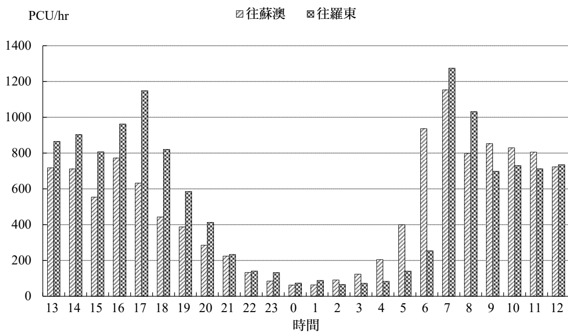
2.5-4 台九線尖峰小時PCU比較圖
