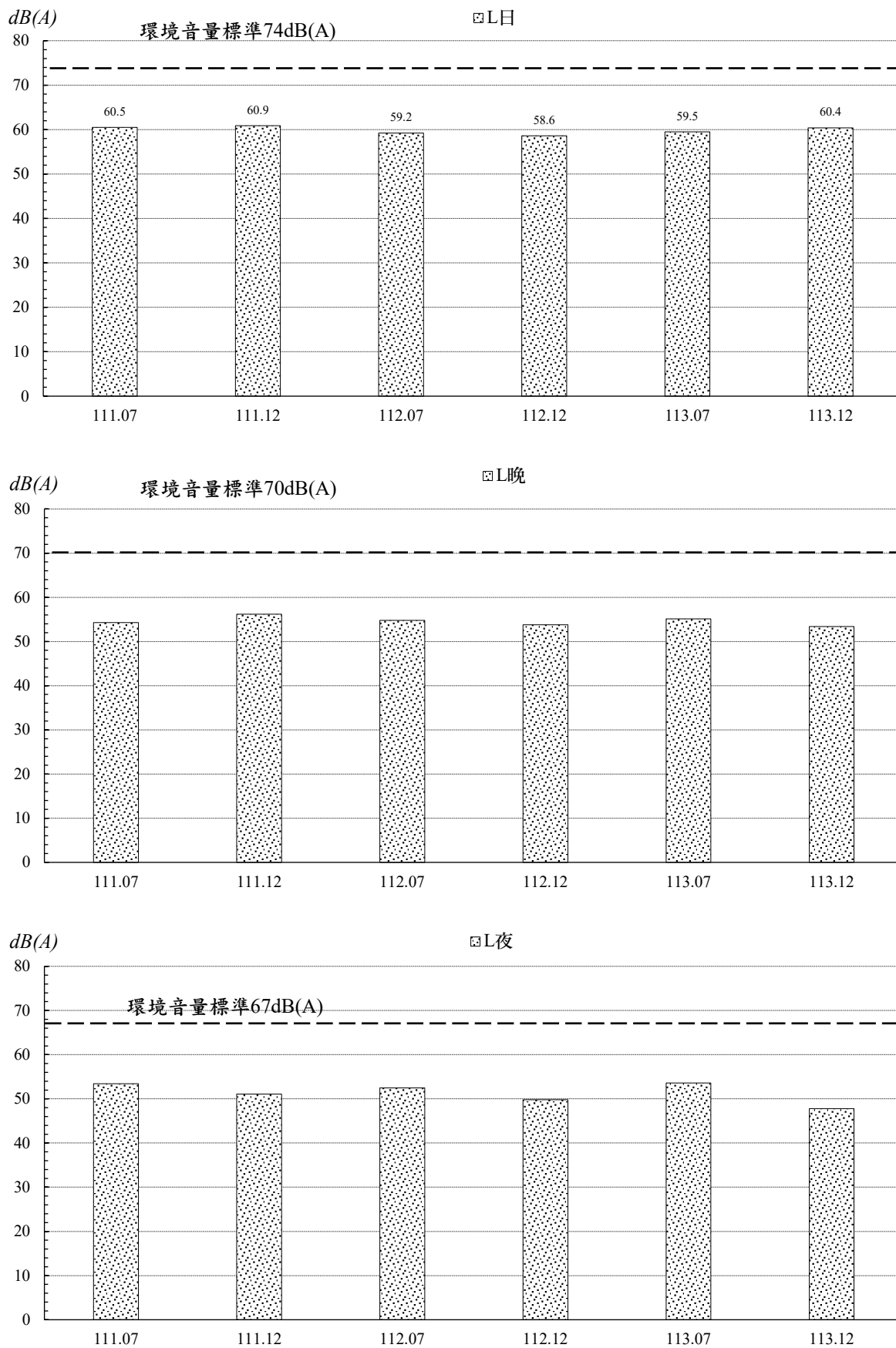
圖2.3-1 永樂路噪音監測值與標準比較圖
