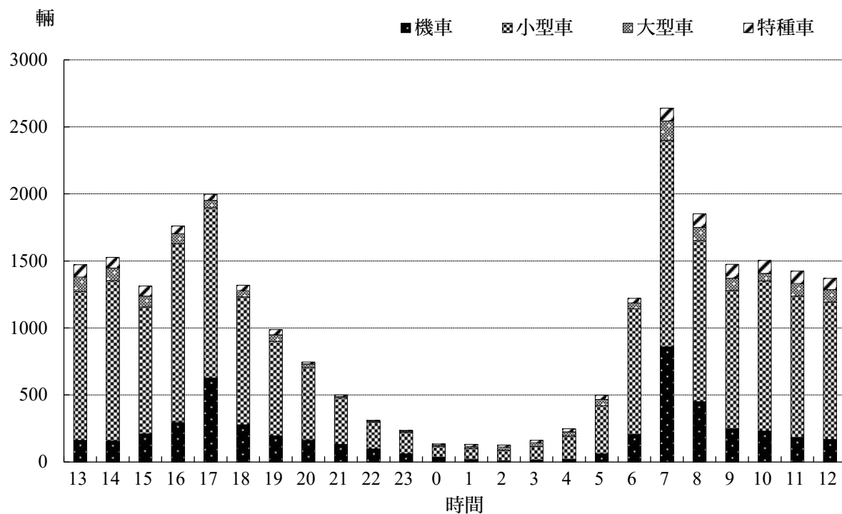
圖 2.5-3 台九線 24 小時單位車輛組織柱狀圖
