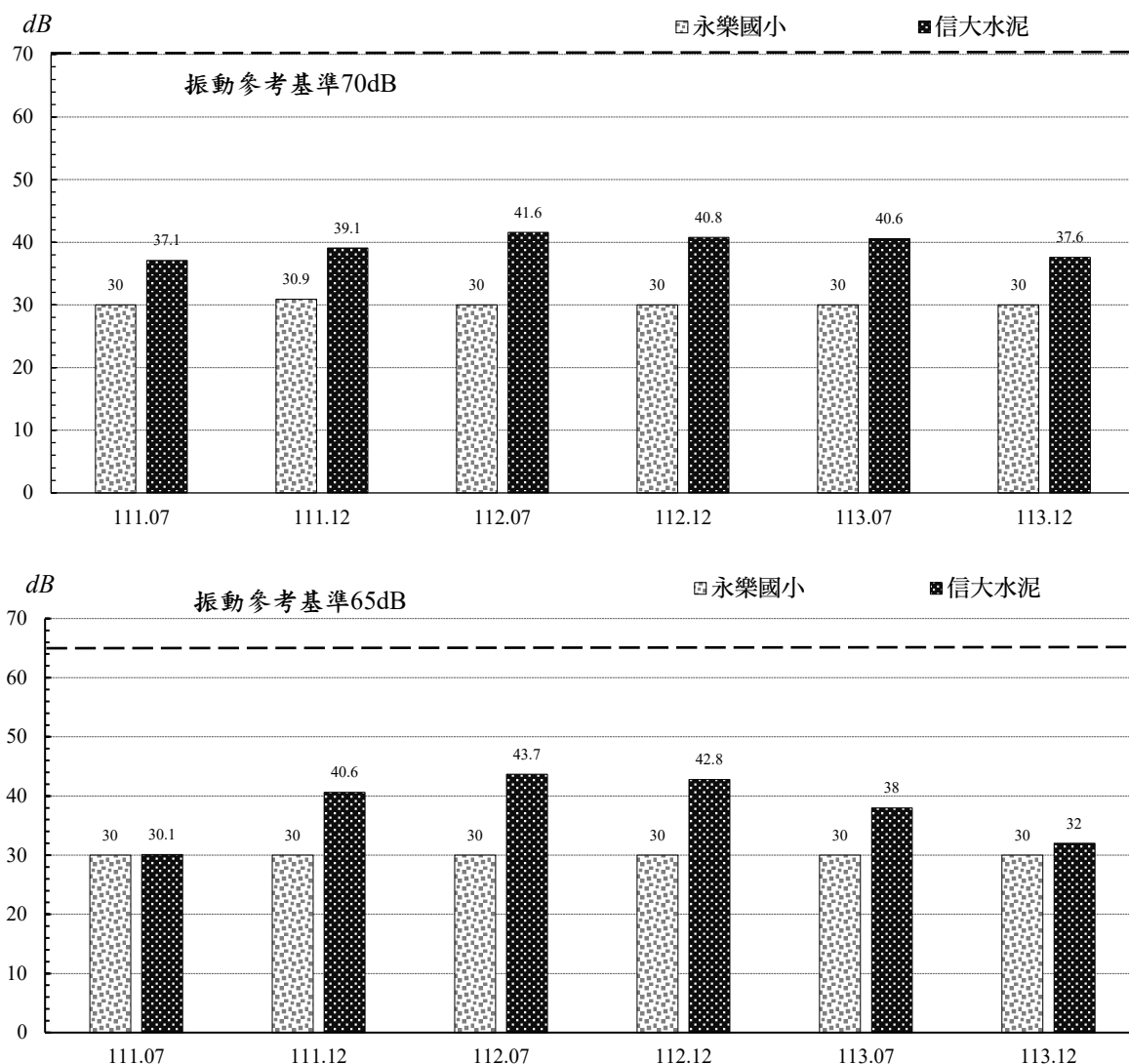
圖2.4-1 振動監測值暨基準值比較圖
